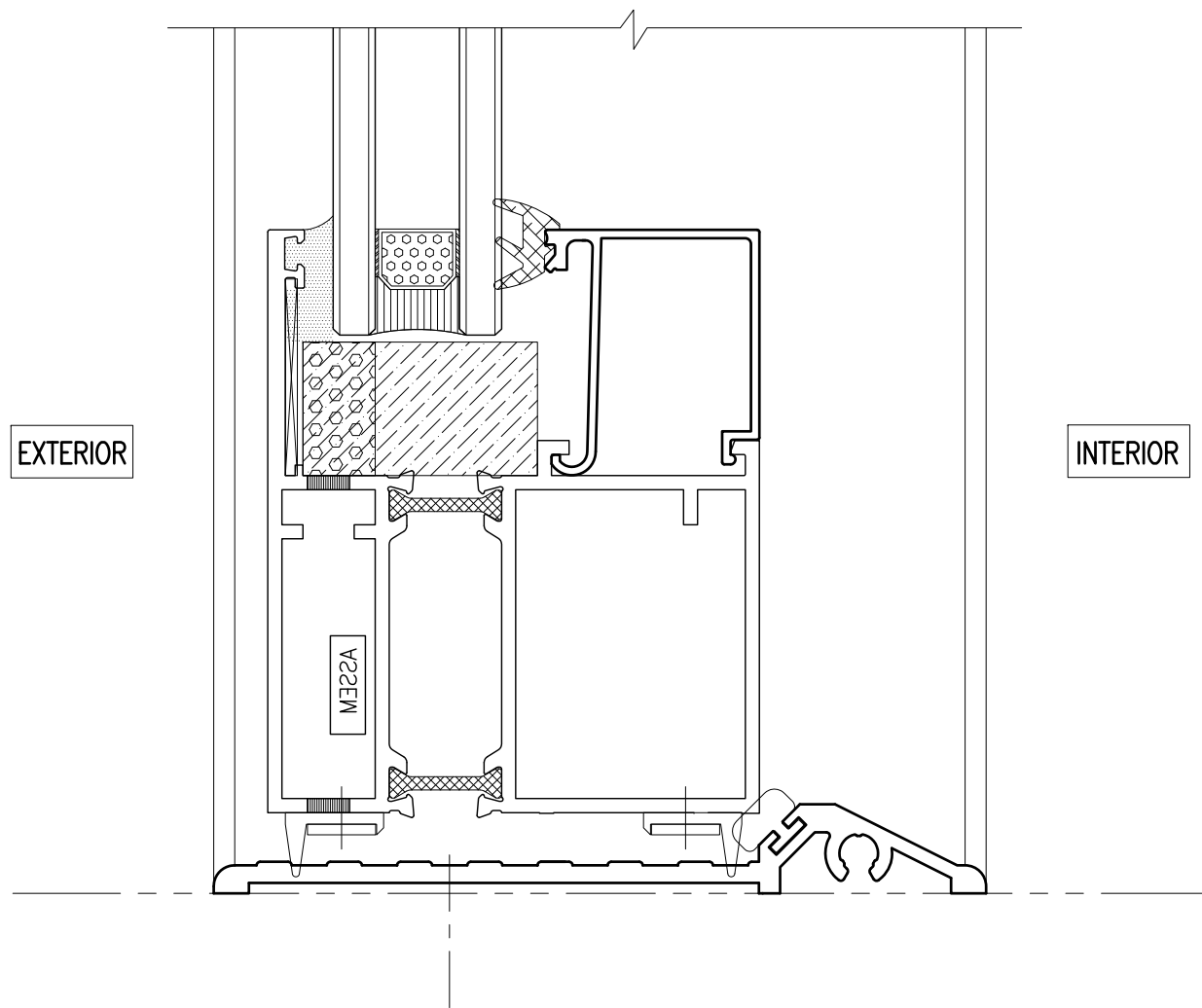
① ADA Door – Inswing
