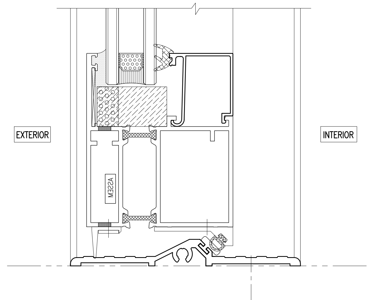
② ADA Door – Outswing
