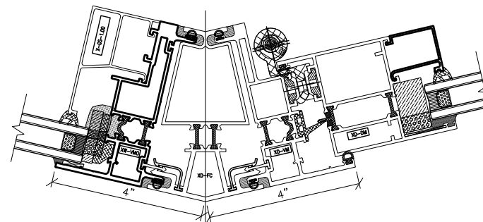
6 DOOR HINGE / FIXED GLASS
