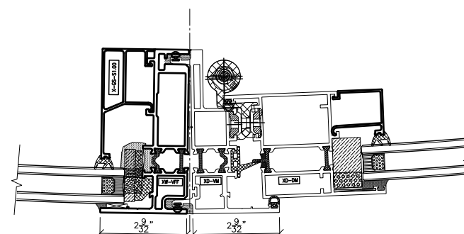
6 DOOR HINGE / FIXED GLASS
