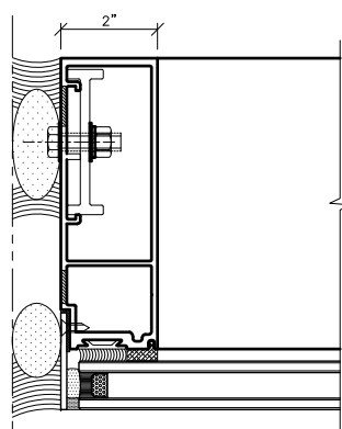
7 Jamb Mullion
